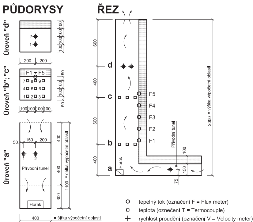
Obrázek 2: schéma rozmístění a označení měřících zařízení
