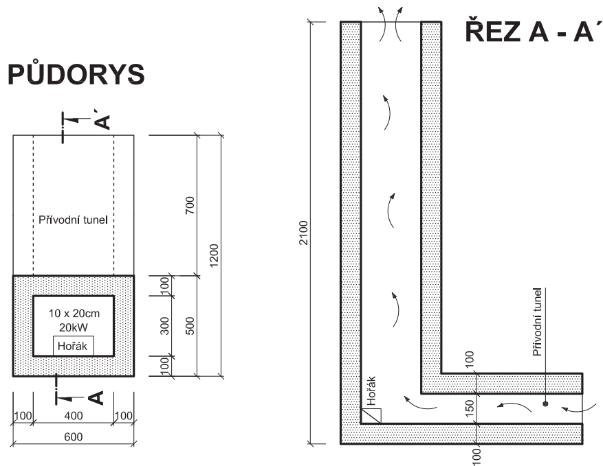
Obrázek 1: model průběžné nehořlavé šachty (fáze 1 - varianta 1)
